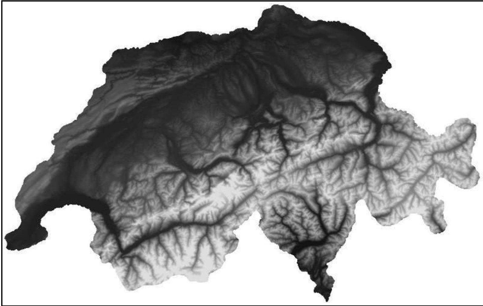
Рис. 11. ЦМР, построенная специалистами SARMAP (разработчиками SARscape) по данным тандемной интерферометрической съемки со спутников ERS-1 и ERS-2 в конце 1990-х годов. Используемые функции: фокусировка радиолокационных голограмм, интерферометрическая обработка с получением на выходе ЦМР, создание мозаики выходных ЦМР, вырезка по векторному файлу государственной границы Швейцарии [3].
