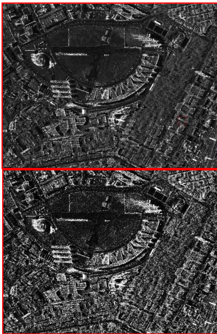
Рис. 9. Исходная (сверху) и фильтрованная мультитемперенным фильтром (снизу) амплитуда радарного снимка TerraSAR-X (Infoterra GmbH). Использованы функции импорта, некогерентного накопления, корегистрации и мультитемперенной фильтрации (Совзонд, 2010).
