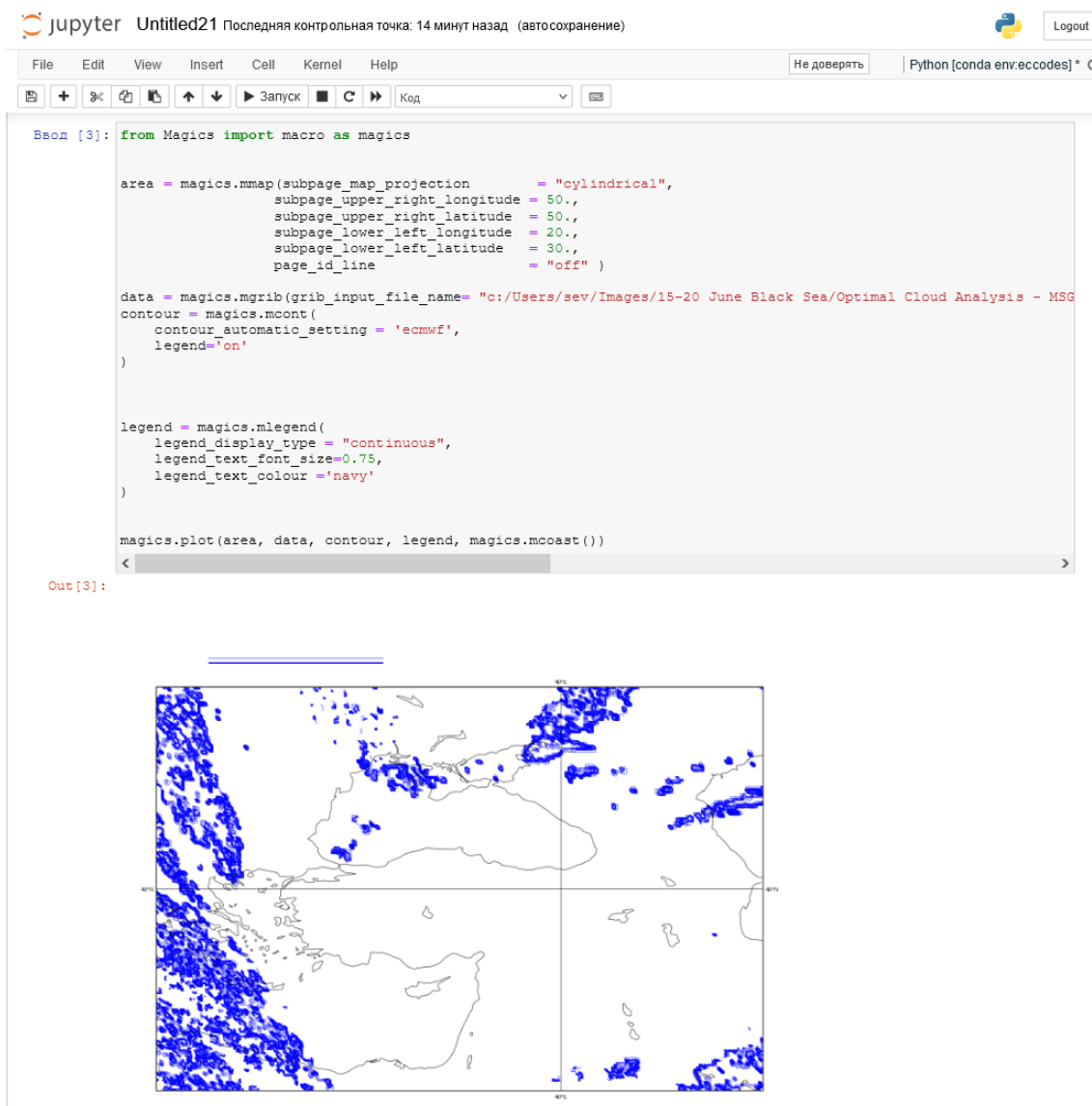
Рис. 3. Веб-интерфейс пакетов eccodes и Magics в среде Jupyter Notebook.
