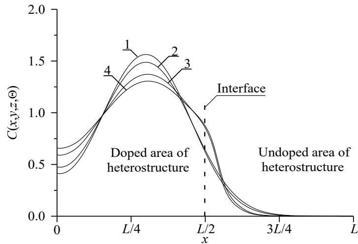
Рис. 2б. Пространственное распределение имплантированной примеси после отжига длительностью \Theta=0,0048(L_x^2+L_y^2+L_z^2)/D_0 (кривые 1 и 3) и \Theta=0,0057(L_x^2+L_y^2+L_z^2)/D_0 (кривые 2 и 4). Кривые 1 и 2 - расчетные распределения в однородной структуре; кривые 3 и 4 - расчетные распределения примеси в двухслойной структуре при условии, что коэффициент диффузии примеси легированном слое больше, чем в соседнем
