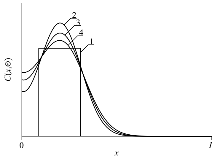
Рис.4б. Пространственные распределения примеси в гетероструктуре при ионном легировании. Кривая 1 - требуемое идеализированное распределение при меси. Кривые 2-4 - реальные распределения примеси в различные моменты времени (увеличение номера кривой соответствует увеличению длительности отжига)
