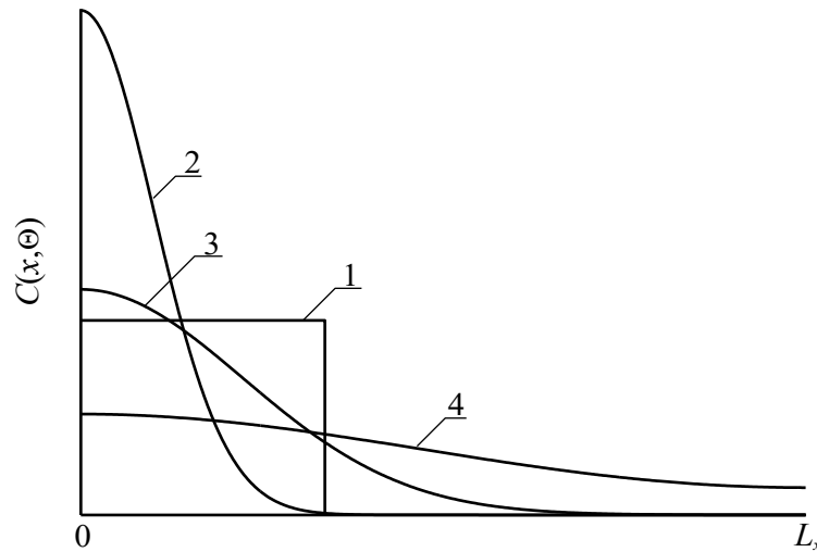
Рис.4а. Пространственные распределения при меси в гетероструктуре при диффузионном легировании. Кривая 1 - требуемое идеализированное распределение при меси. Кривые 2-4 - реальные распределения примеси в различные моменты времени (увеличение номера кривой соответствует увеличению длительности отжига)
