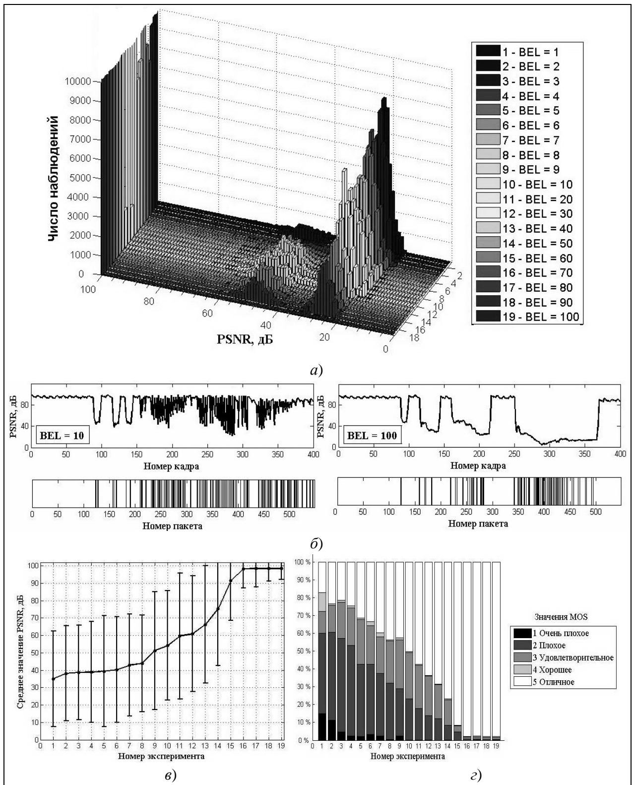
Рис. 4. Значения показателей качества видеопоследовательности при PER = 1 \cdot 10^{-3} и различных значениях BEL беспроводного канала: а – гистограммы распределения значения PSNR; б – значения PSNR и распределение RTP/UDP пакетов (черные участки соответствуют потерянным пакетам) при некоторых значениях BEL; в – девиация качества по средним значениям PSNR; г – градация качества по значениям MOS
